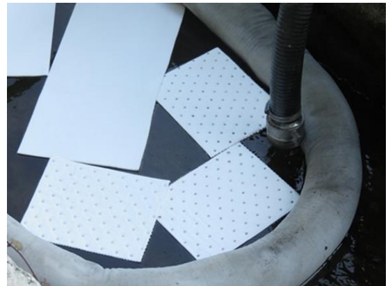
吸着型オイルフェンスの設置と吸引車による油回収
